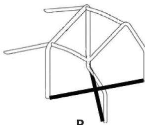
P Croce a pavimento dwg. 253-31
