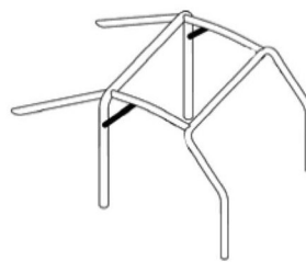
K Rinforzi su arco posteriore dwg. 253-31
