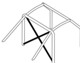
N Croce su arco principale dwg. 253-7
