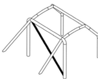
I Diagonale su arco principale dwg. 253-5
