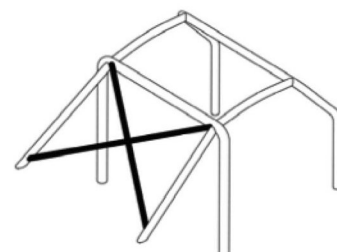
Q Croce su braccia posteriori dwg. 253-21
