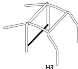
H3 Traversa attacco cintura dwg. 253-30
