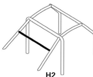
H2 Traversa attacco cintura dwg. 253-28
