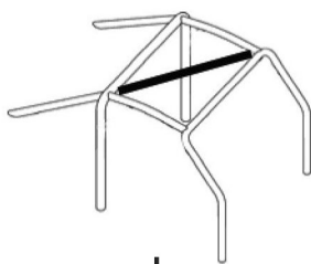
J Diagonale su tetto
