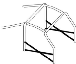
A1 Rinforzo porta a croce dwg. 253-9
