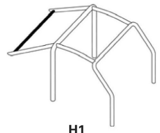
H1 Traversa attacco cintura dwg. 253-18
