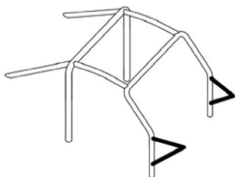
C Attacco ai duomi anteriori dwg. 253-25
