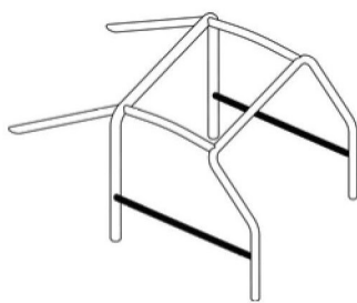
A2 Rinforzo porta semplice dwg. 253-8
