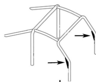
L Rinforzi in lamiera piegature arco anteriore
