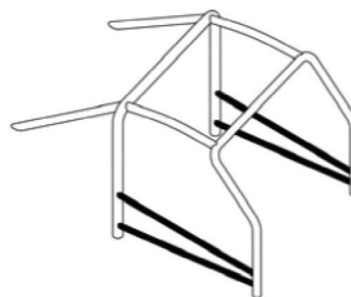
A3 Rinforzo porta doppio dwg. 253-11
