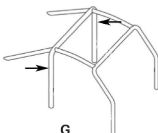
G Attacchi dell'arco posteriore sul montante centrale dell'auto
