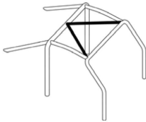
V2 V su tetto
